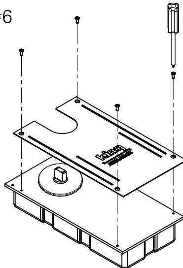
스텐 판 부착 및 볼트 4개 체결
