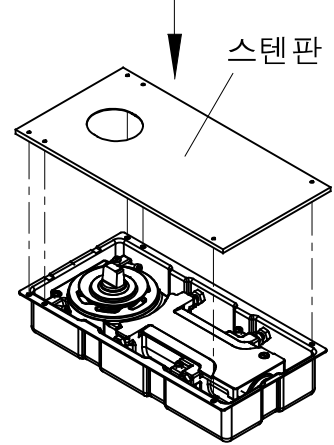
스텐 판 방수커버 부착
