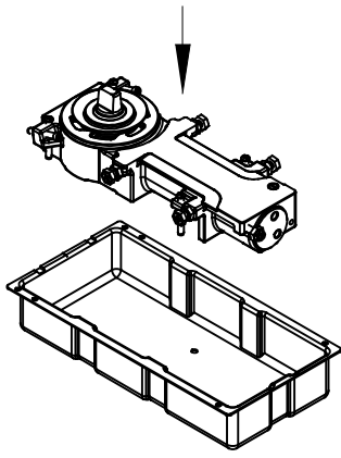
시멘트 케이스에 힌지 부착
