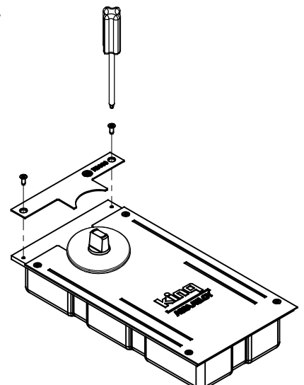
보조스텐 판 부착 및 볼트 2개 체결
