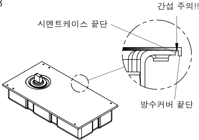
방수커버 끝단과 시멘트케이스 끝단이 서로 간섭되지 않게 부착
