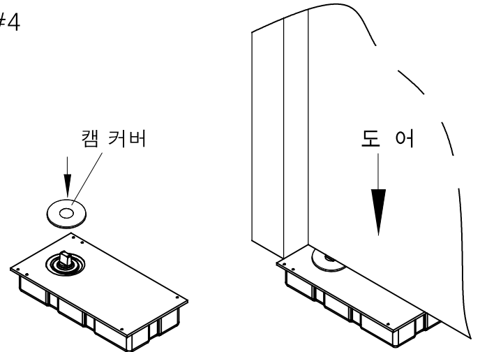
캠커버 부착 및 도어 설치
